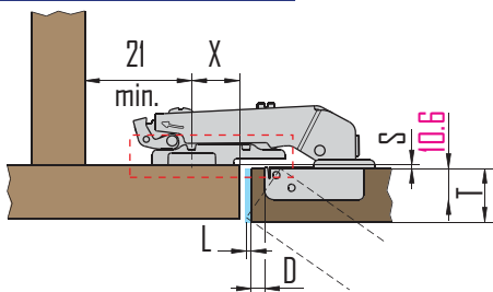
Bisagra Esquina Ciega Brazo Corto
